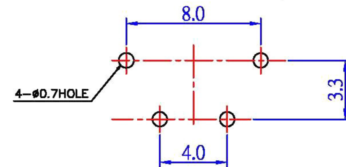
P.C.B LAND PATTERN
